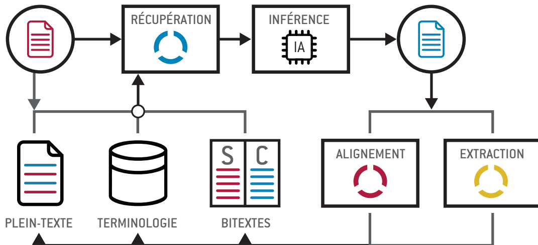
Diagramme logique de TAIGR
